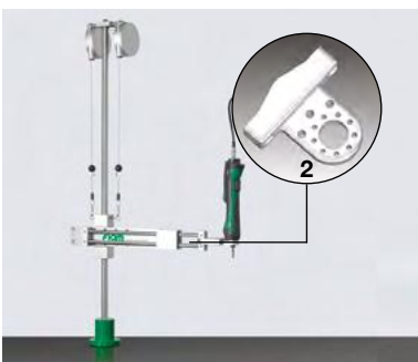
Kartesische Werkzeughalter BCA
